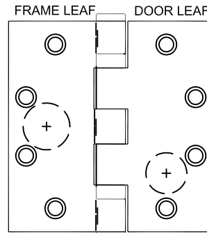
LEFT HAND HINGE
